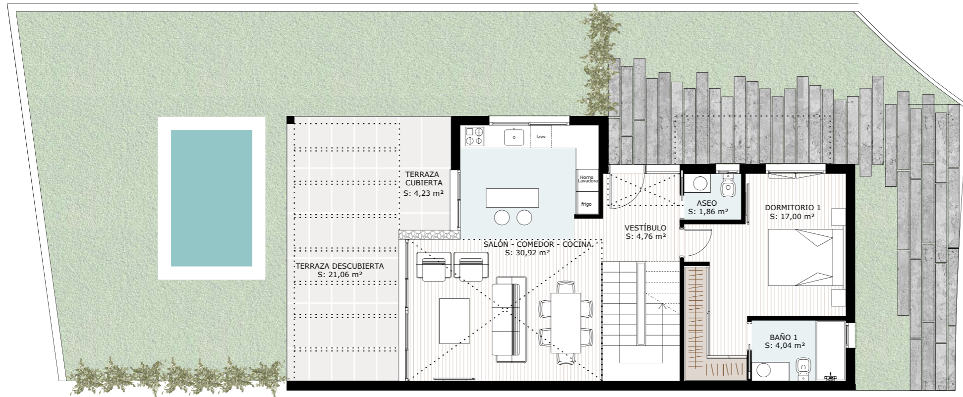
PLANTA BAJA
