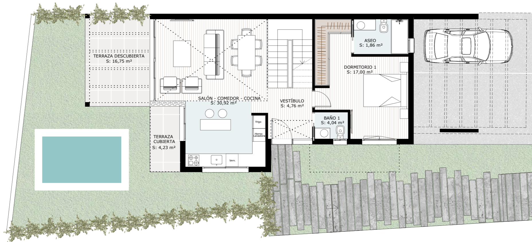
PLANTA BAJA
