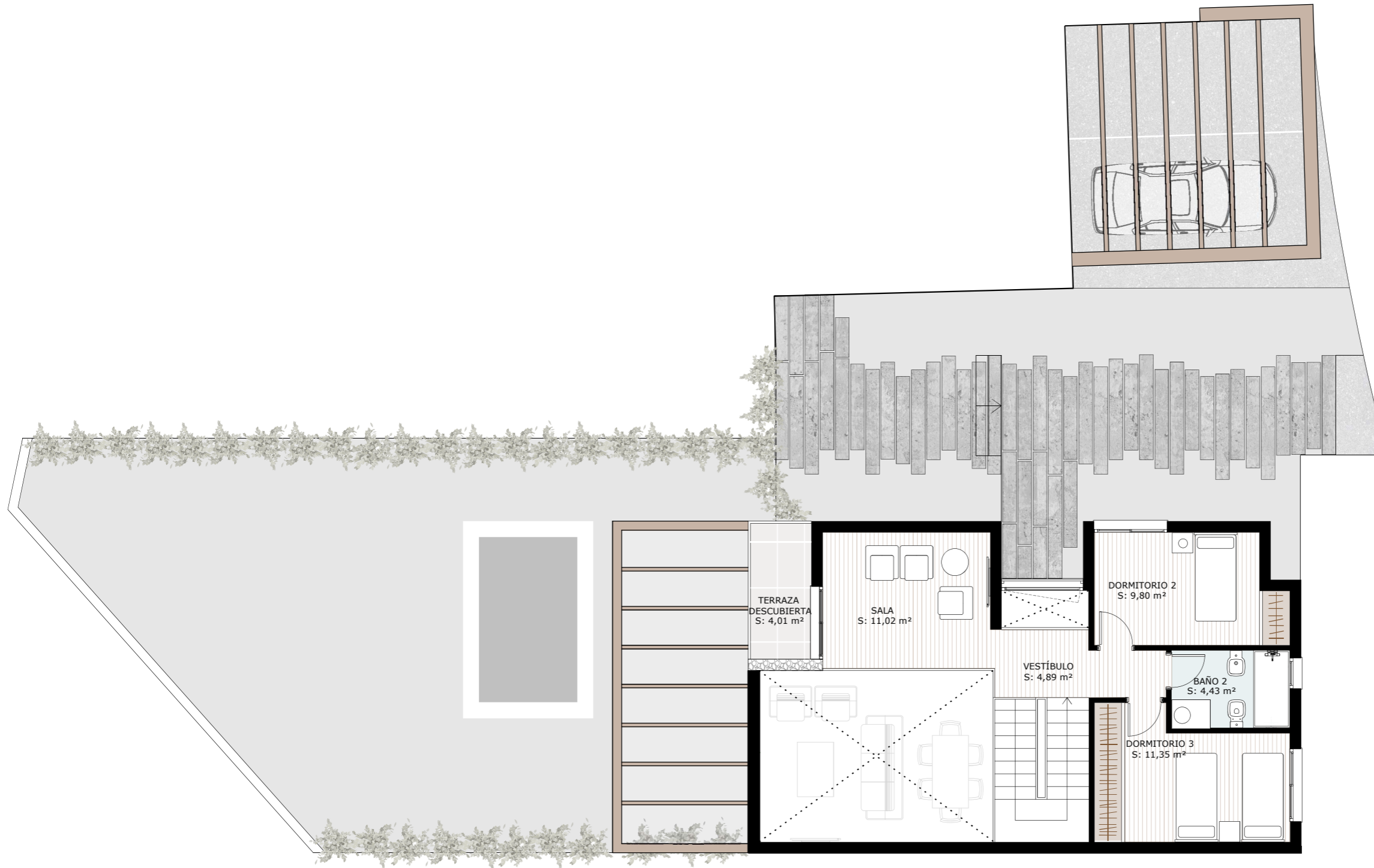
PLANTA PRIMERA
