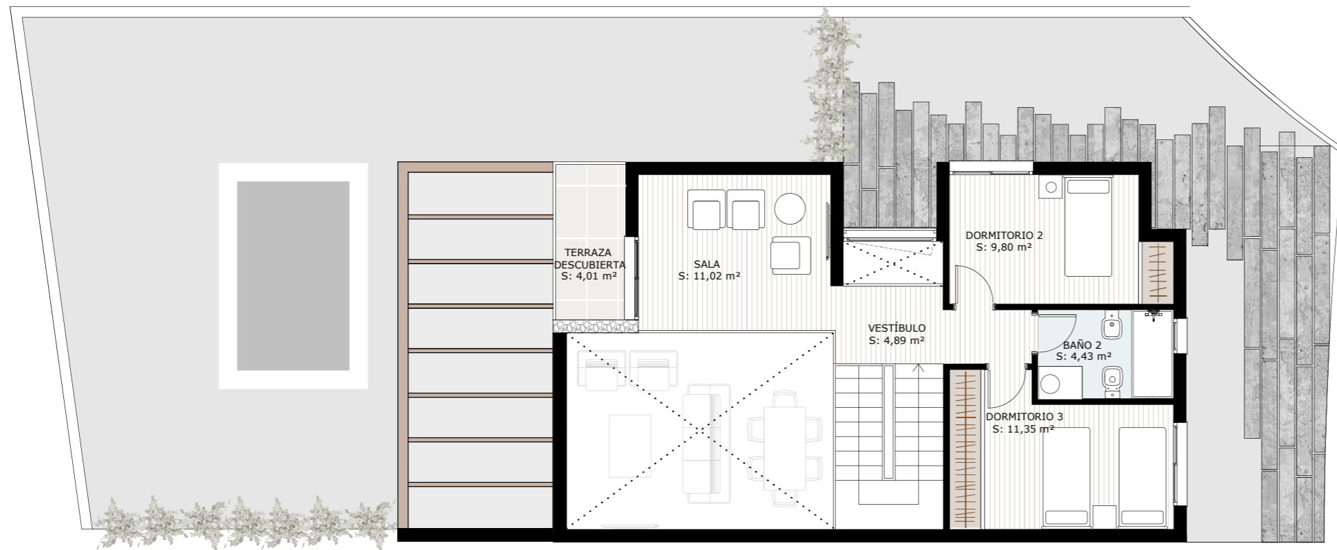
PLANTA PRIMERA
