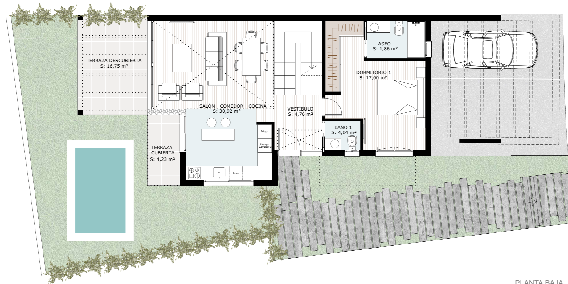
PLANTA BAJA
