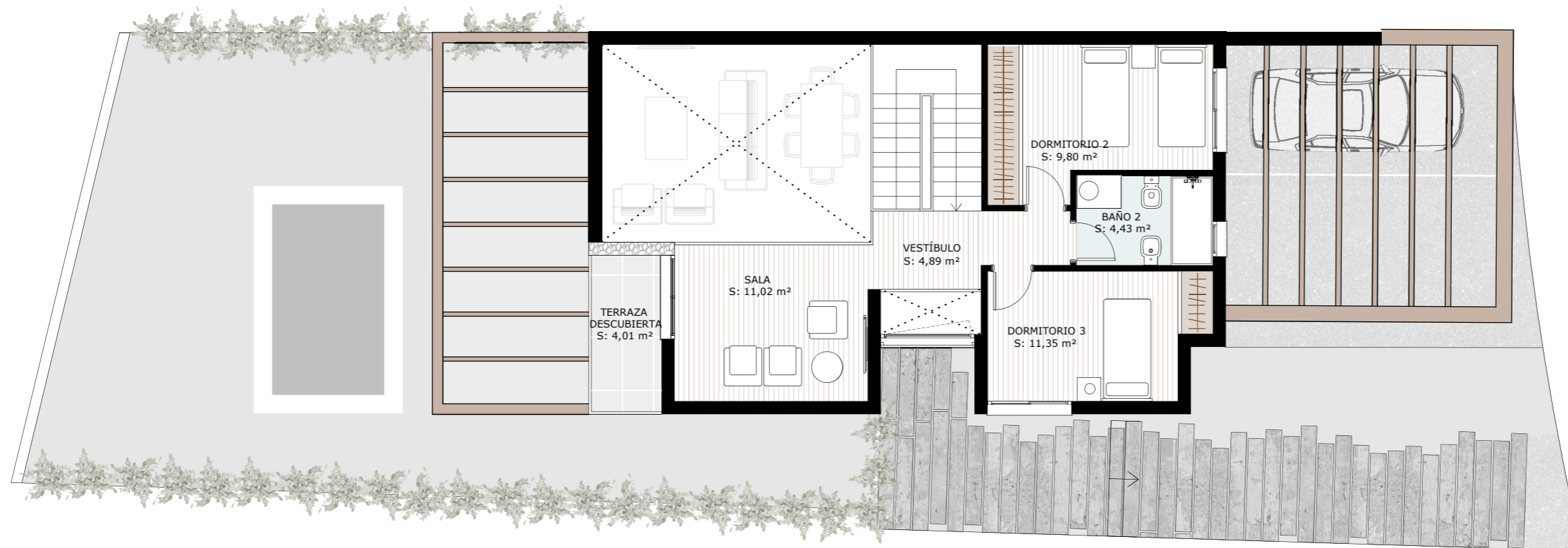
PLANTA PRIMERA
