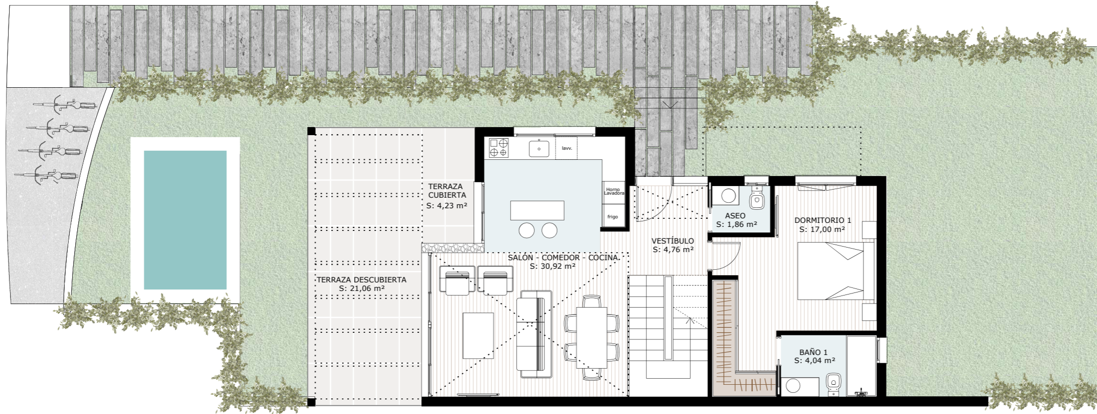
PLANTA BAJA
