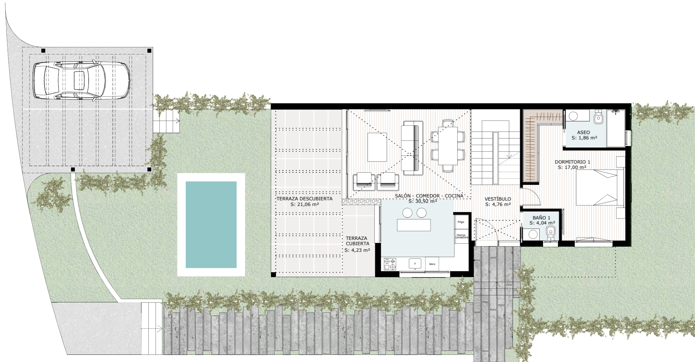
PLANTA BAJA
