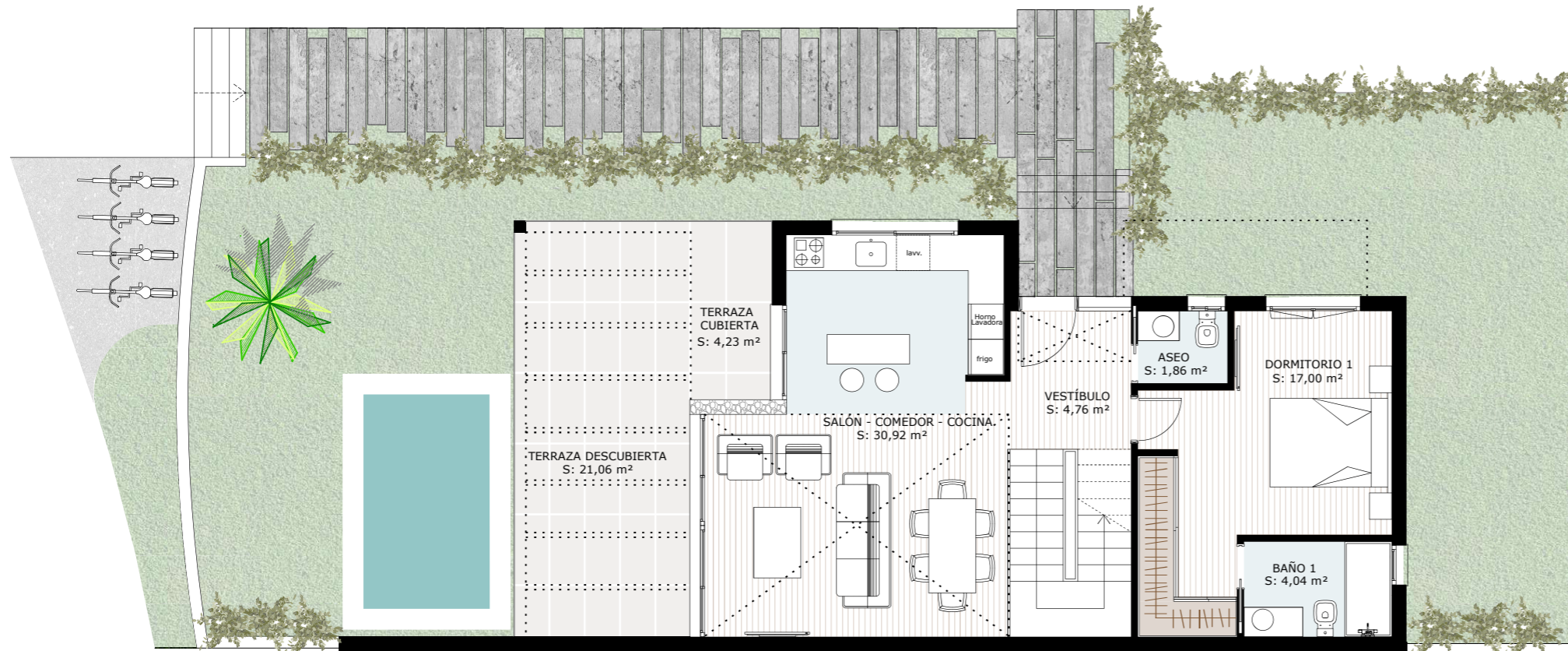
PLANTA BAJA
