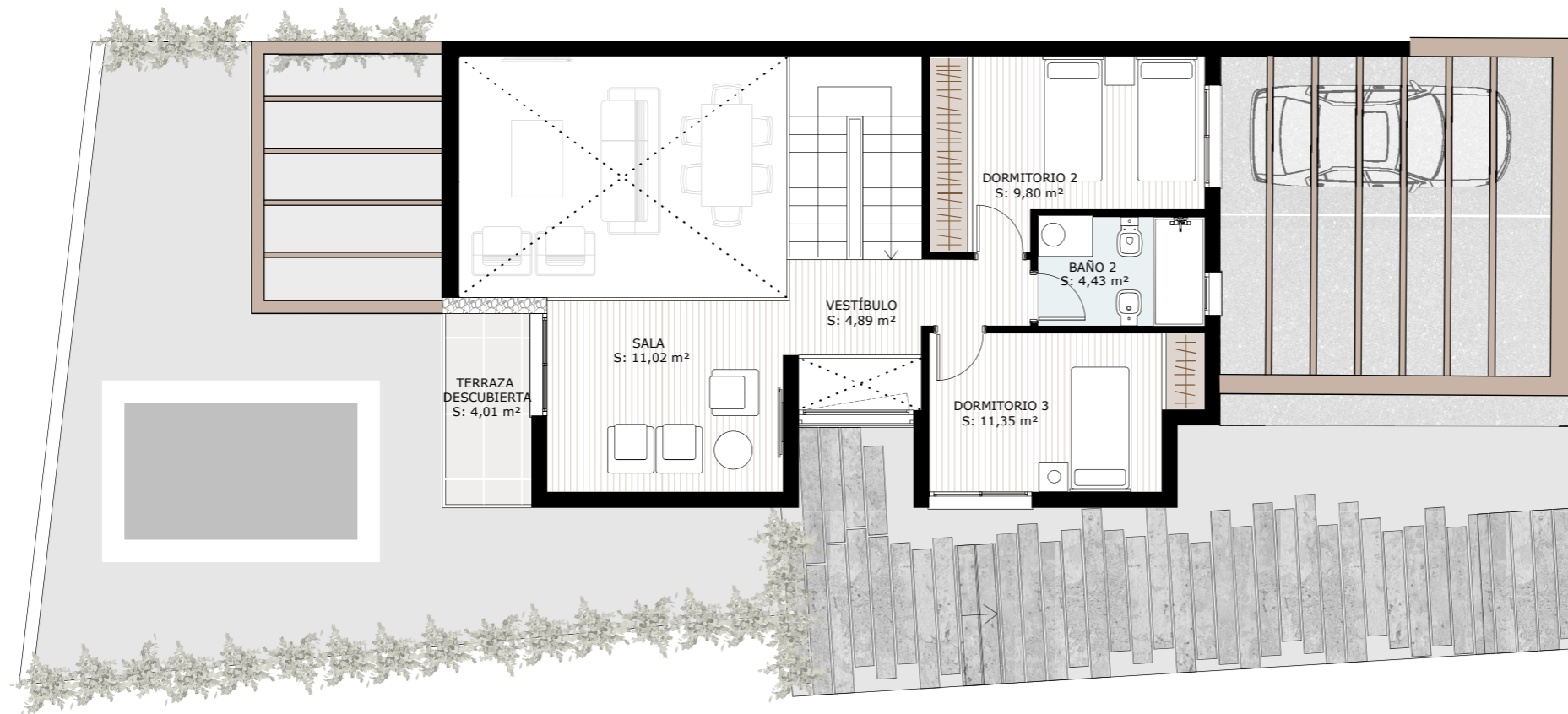
PLANTA PRIMERA
