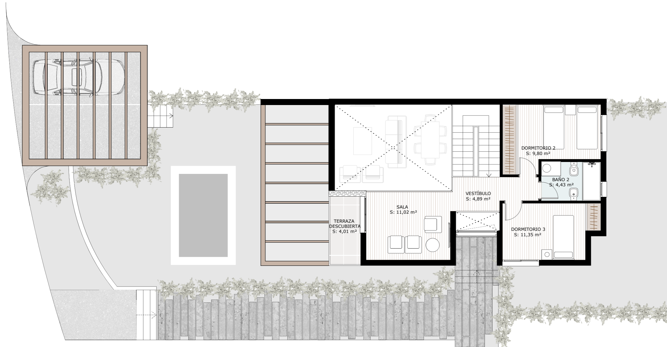
PLANTA PRIMERA
