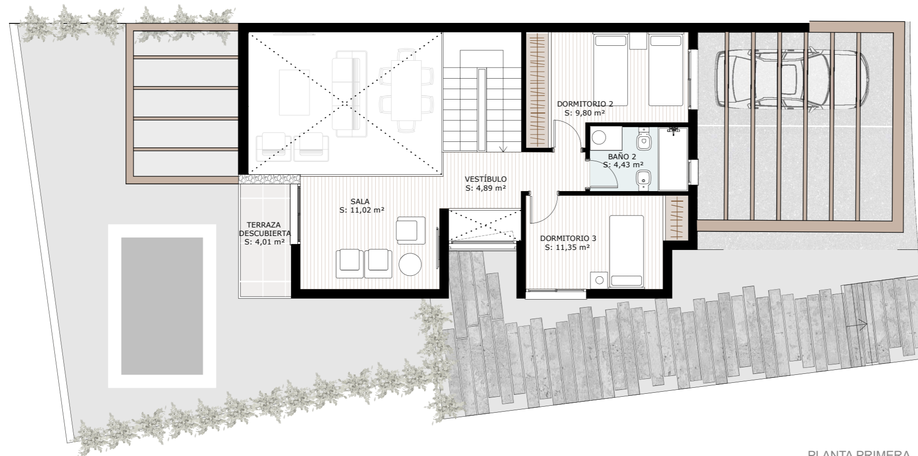
PLANTA PRIMERA
