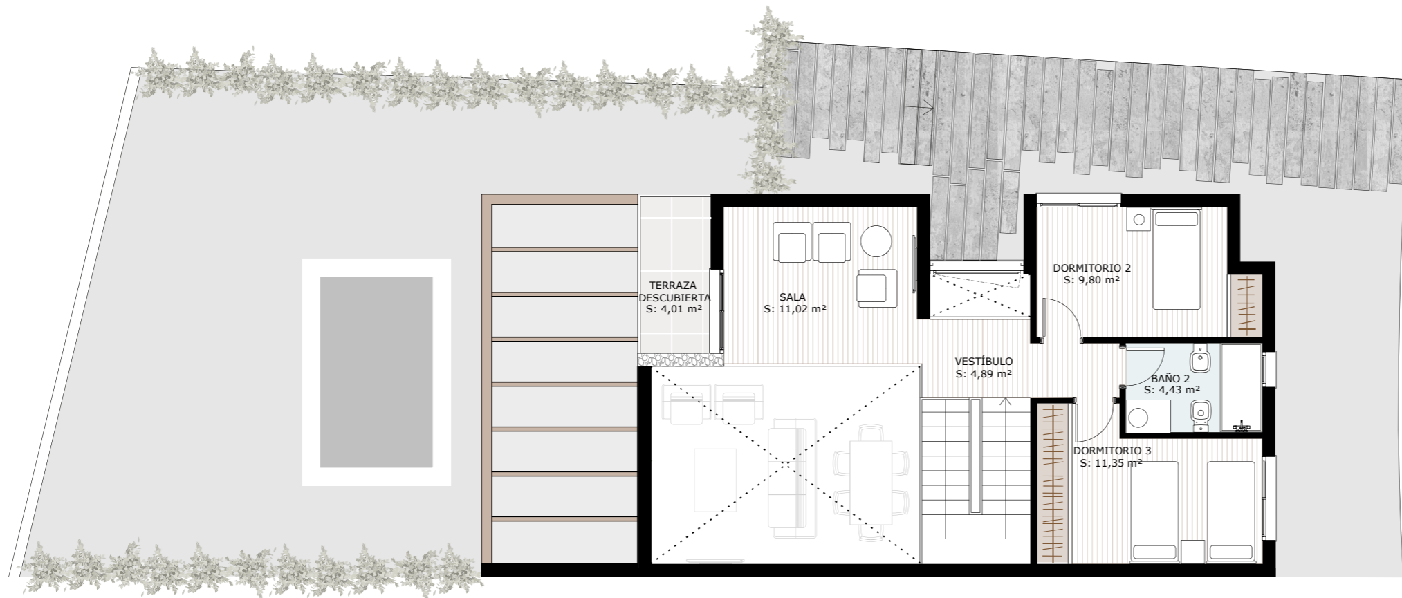
PLANTA PRIMERA
