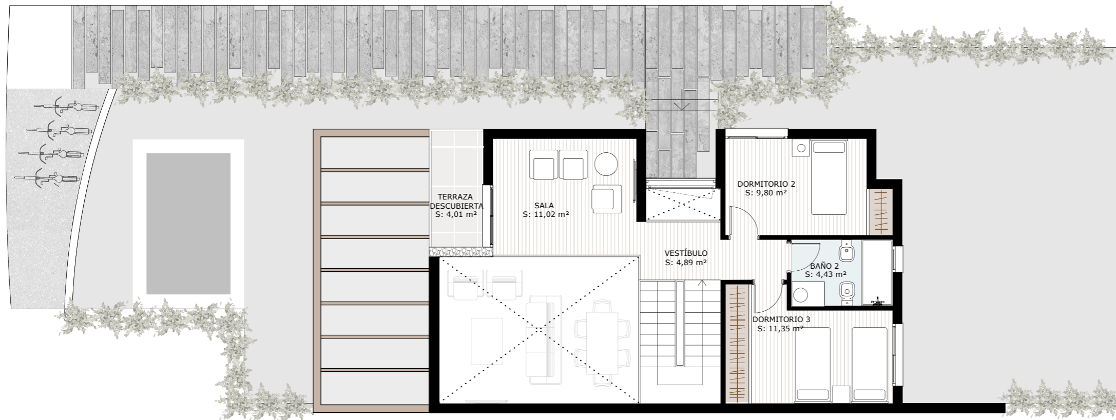
PLANTA PRIMERA
